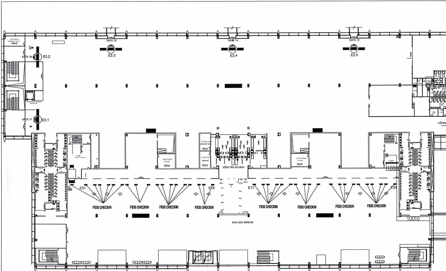
SƠ ĐỒ MẶT BẰNG FIDS TẦNG 2 SÂN H E
